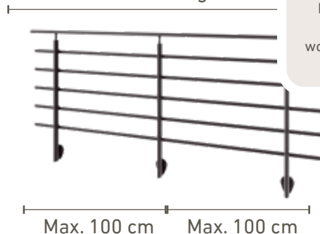
Voorbeeld laterale bevestiging 250 cm lang
